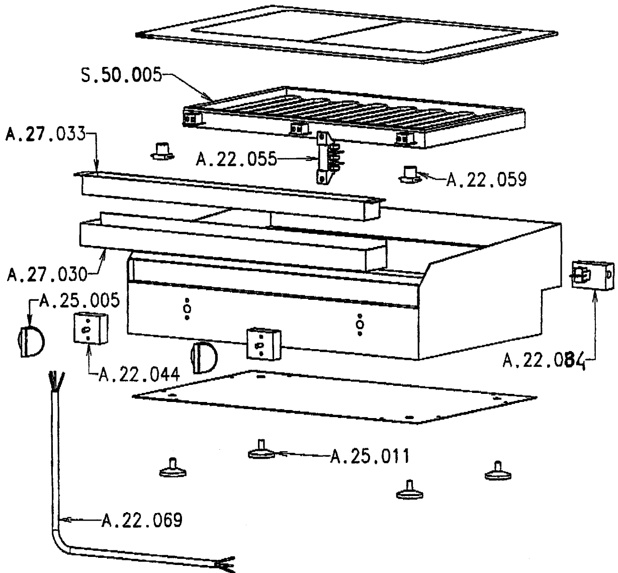
A.90.020 ASSIEME CABLAGGIO ELETTRICO COMPLETO
